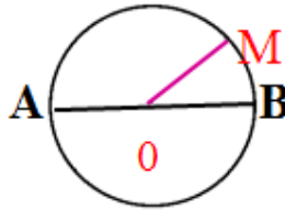
Hình tròn tâm O
